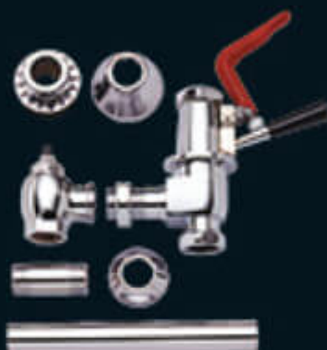
DS-11408 二段式手壓冲水凡而 噴射式、坐式上冲式蹲使用 NT$5000
